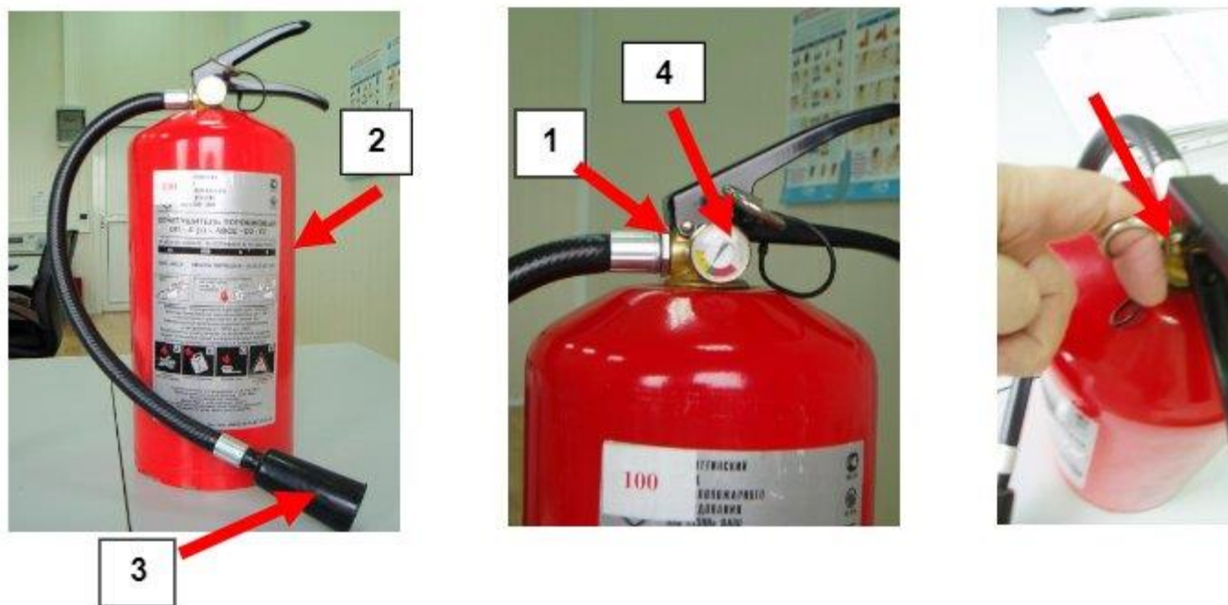
Рис.1. Порошковый огнетушитель типа ОП-4(з)
